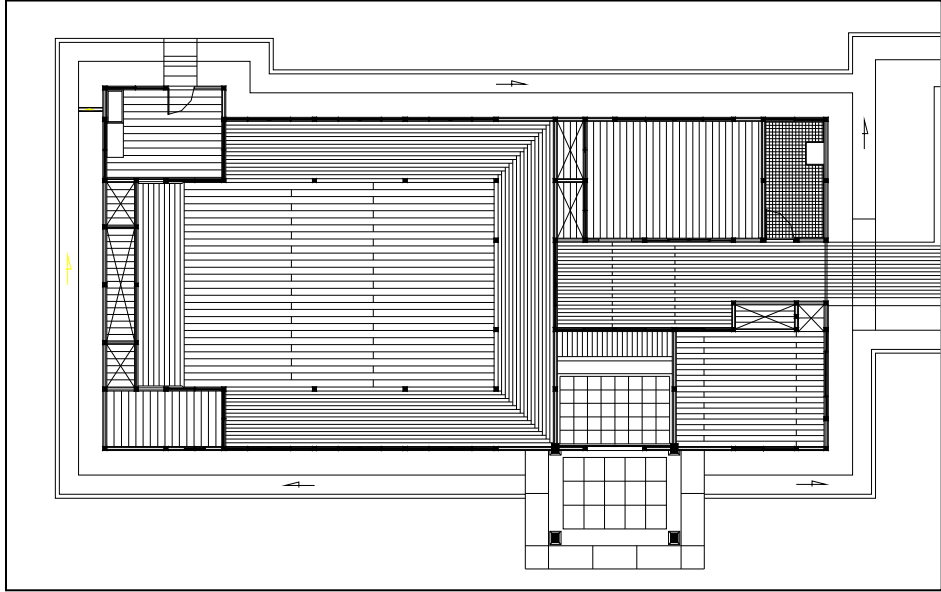
圖 70 齋館平面現況圖
