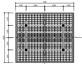
亭水舍屋脊反射平面图
