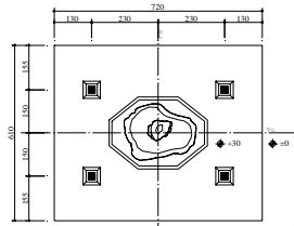
亭水舍平面图
