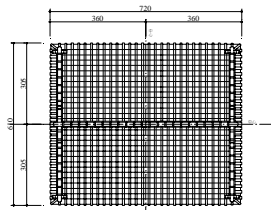
亭水舍屋顶平面图
