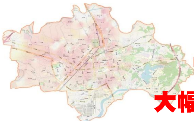
嘉義市108年上半年PM 2.5 感測濃度熱力圖
