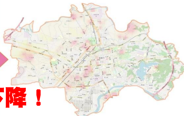
嘉義市111年上半年PM 2.5 感測濃度熱力圖
