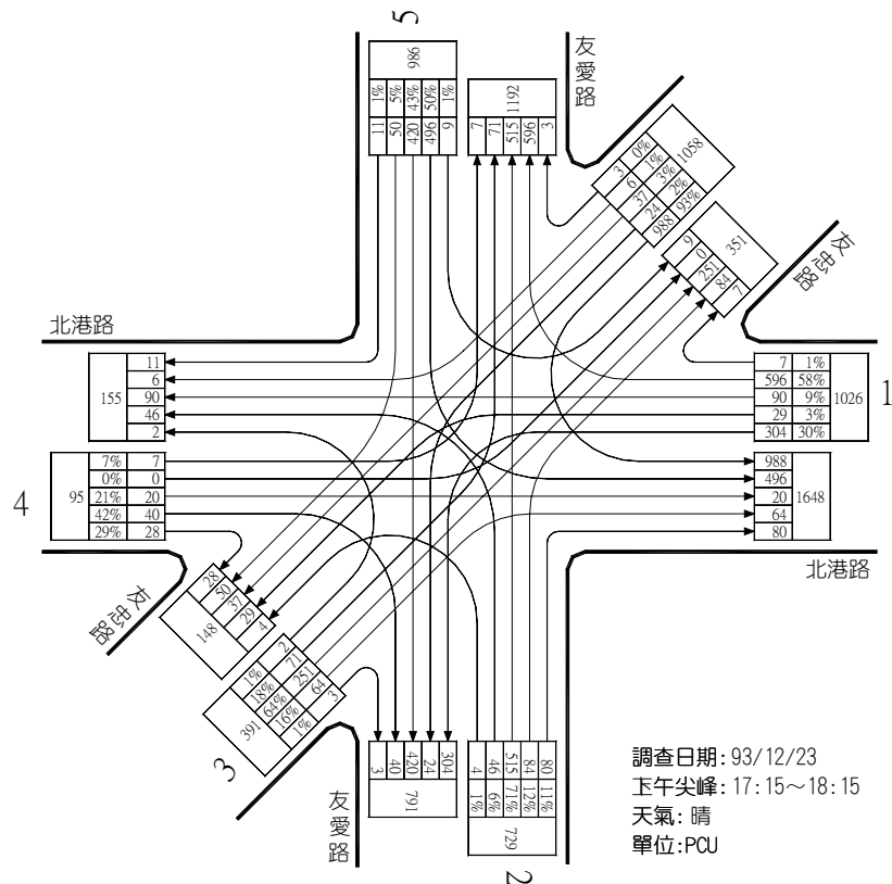
圖 3 北港路/友愛路/友忠路尖峰小時路口轉向交通量示意圖
