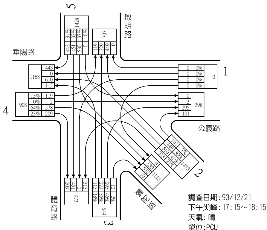
圖 15 公益路/彌陀路/啟明路尖峰小時路口轉向交通量示意圖
