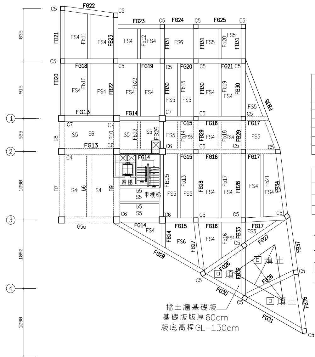
基礎層結構平面圖 S:1/200
