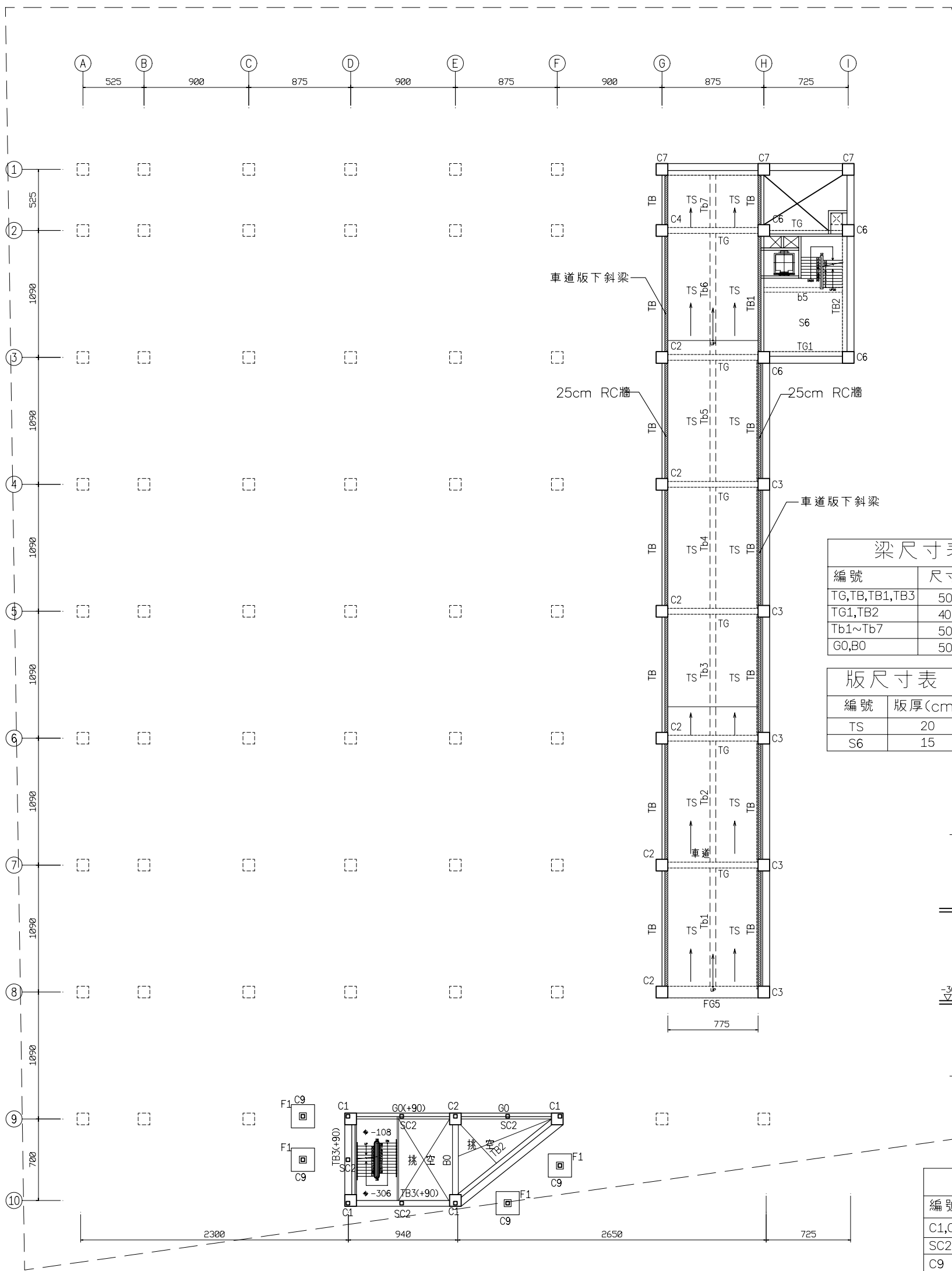
夾層結構平面圖 S:1/200
