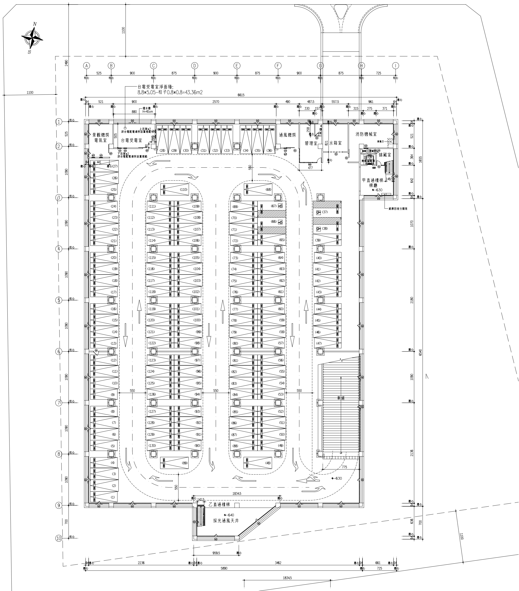
地下一樓平面圖 S:1/200
