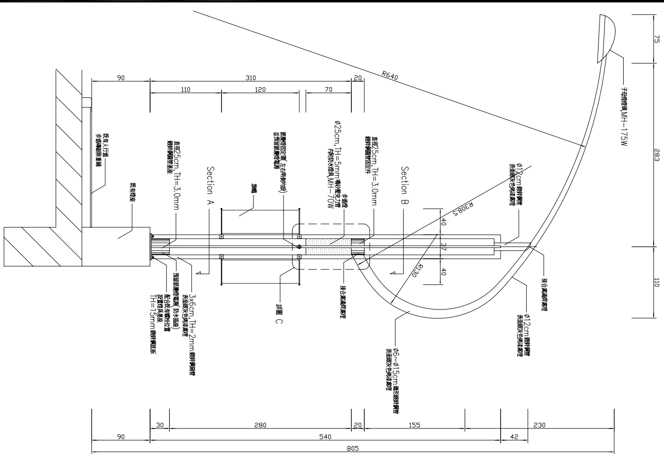
牛稠溪橋路登立面詳圖
