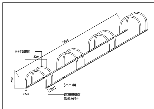
自行車停放架
