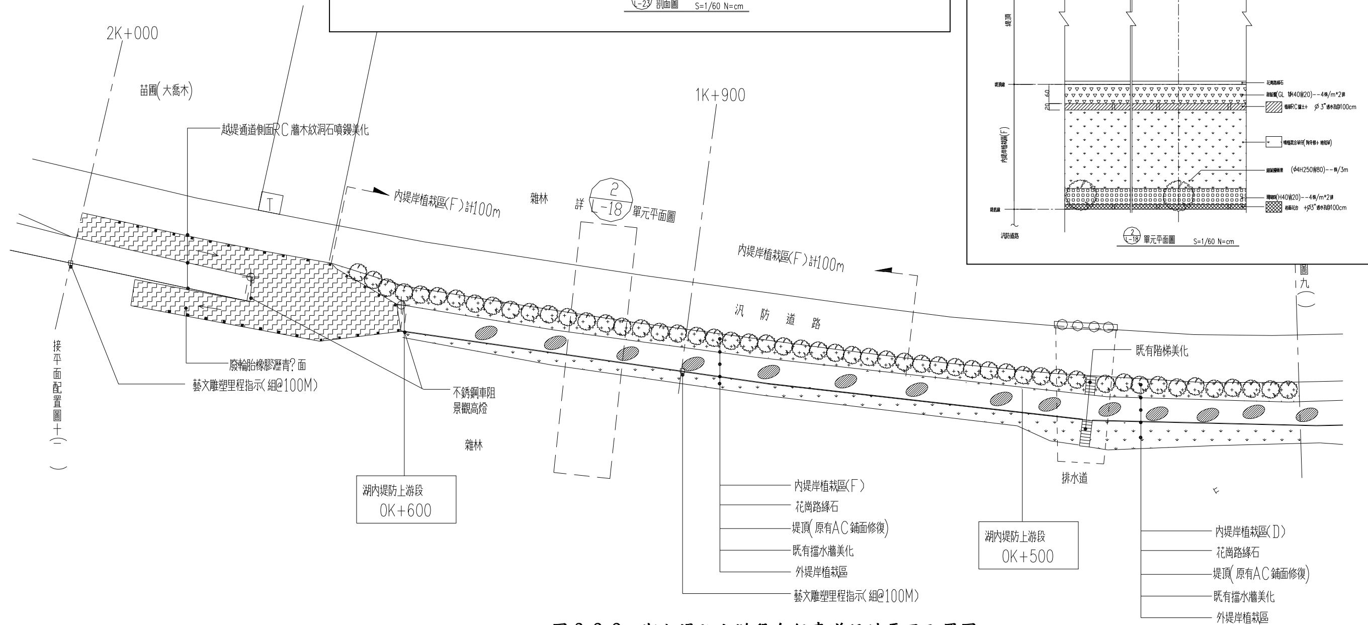
圖 3-2-2 湖內堤防上游段自行車道設計平面配置圖
