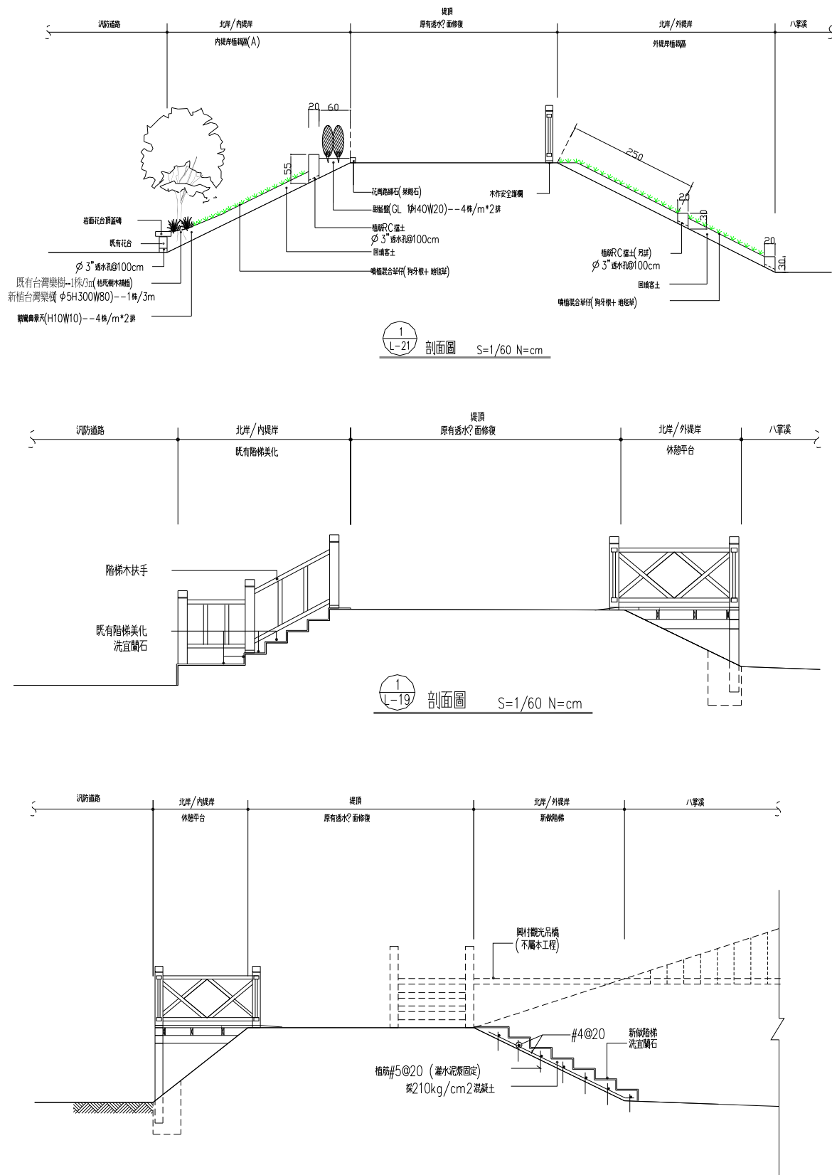
圖 2-2-5 吳鳳堤防段 (0k+000~1k+300) 立面配置構想說明圖
