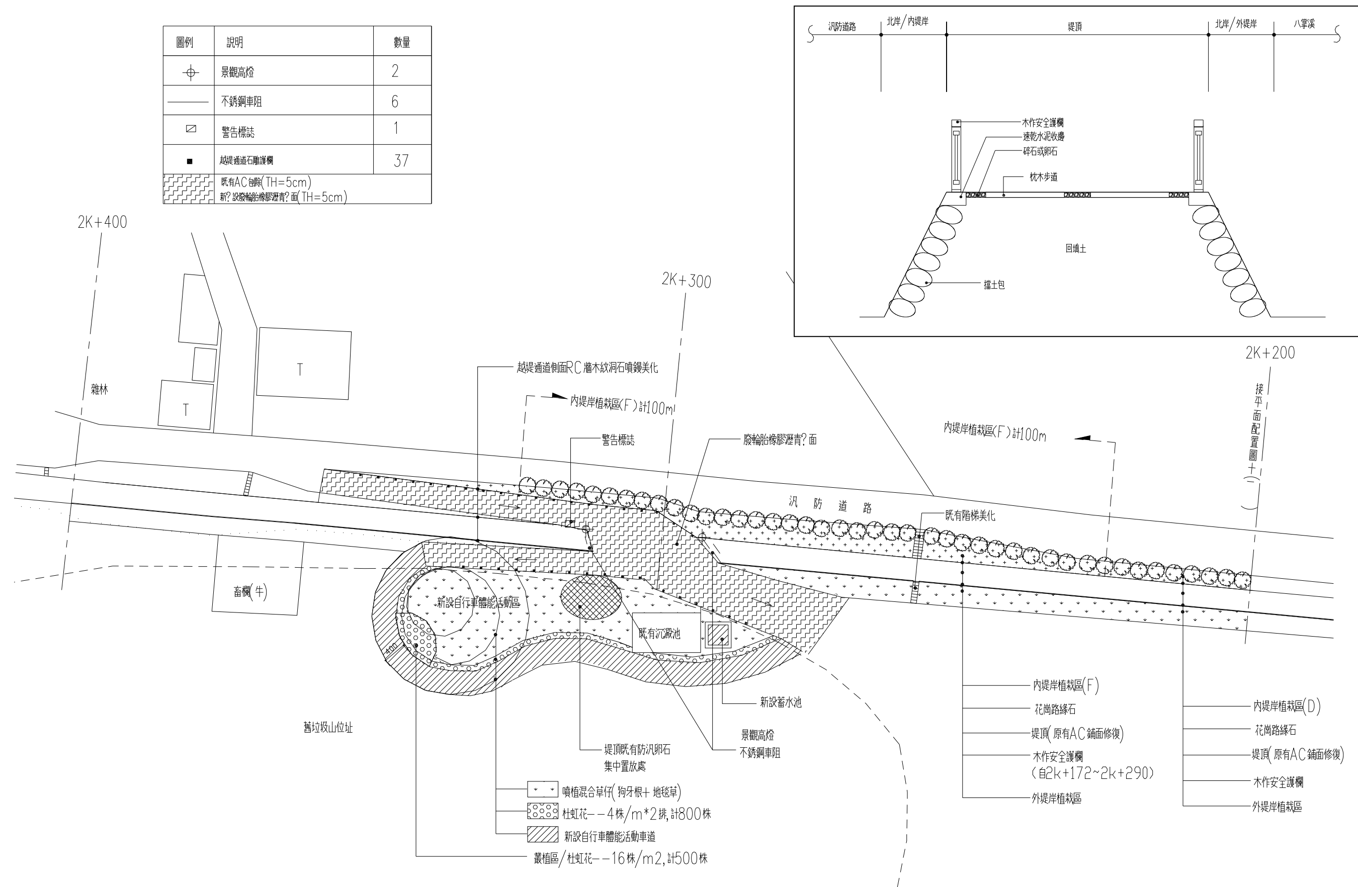
圖 3-2-3 湖內堤防下游段自行車道設計平面配置圖
